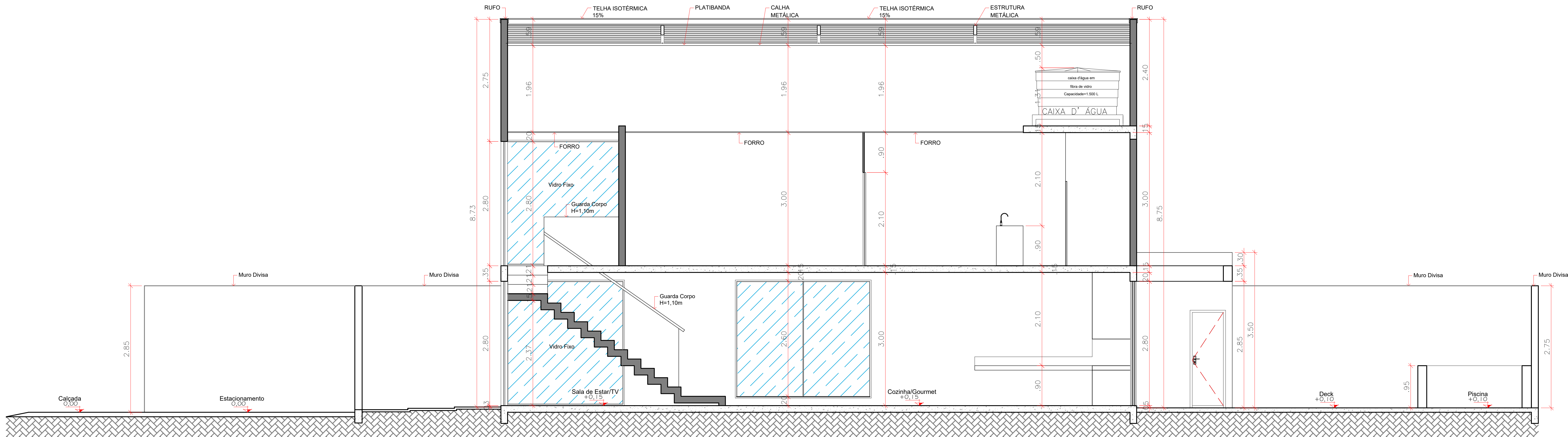
CORTE - "A-A"
