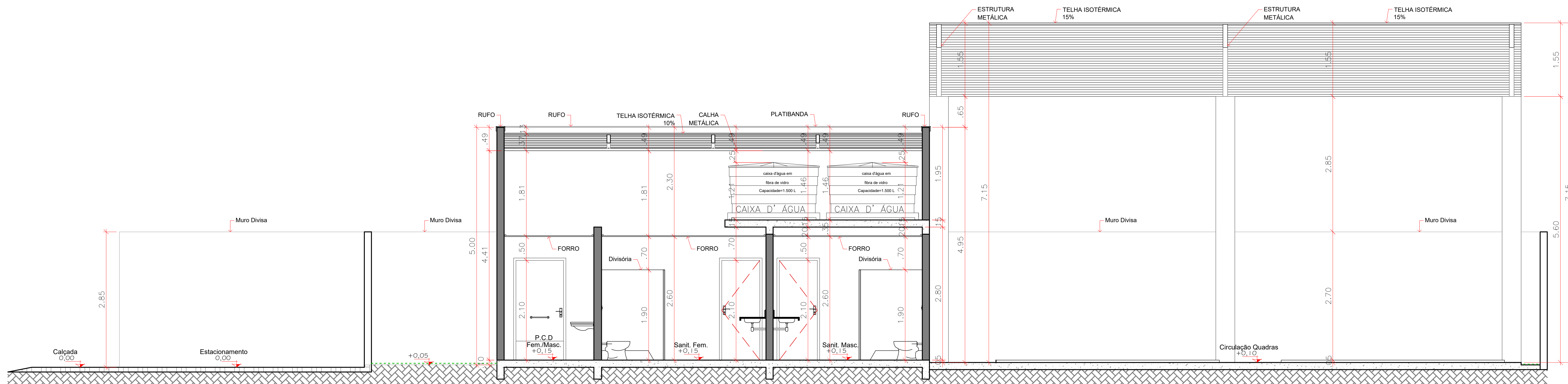
CORTE - "C-C"
