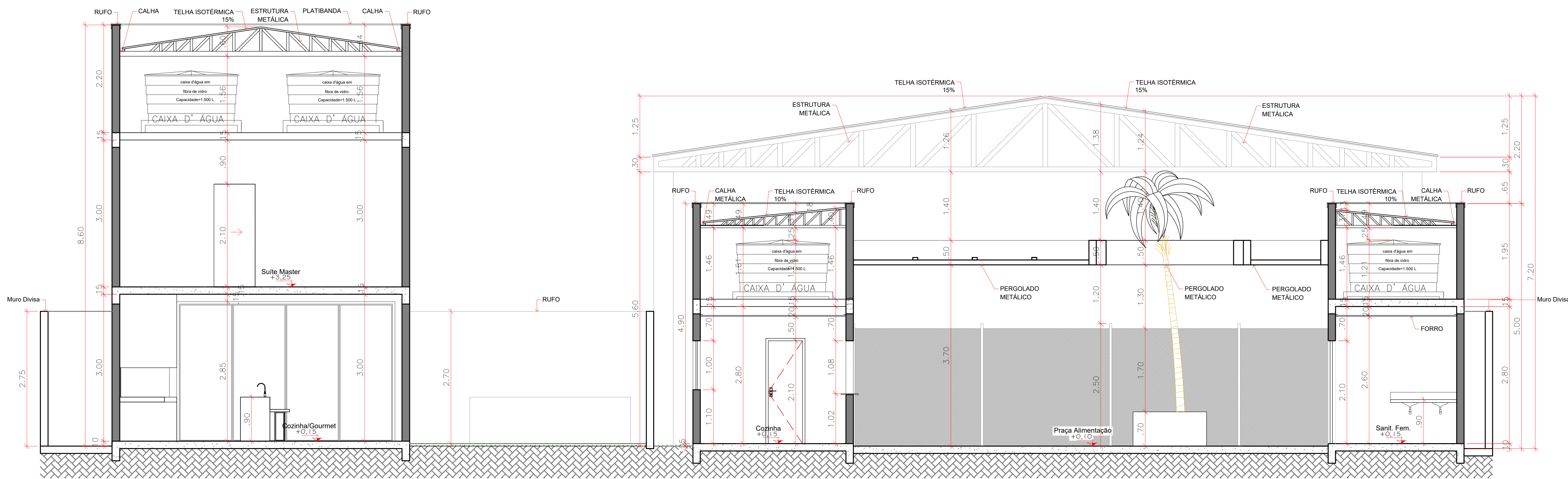
CORTE - "B-B"
